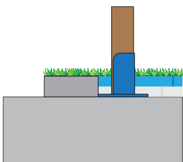
MONTAJE VALLA INTERIOR TORNILLOS OCULTOS
