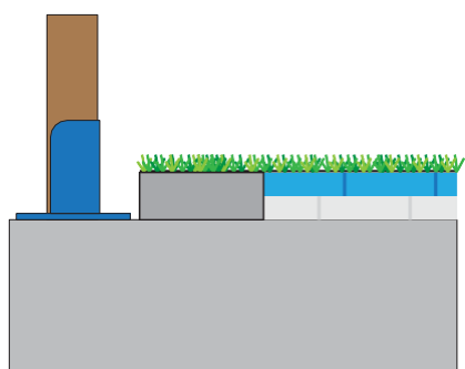
MONTAJE VALLA EXTERIOR TORNILLOS VISTOS POSIBILIDAD EMBELLECEDORES
