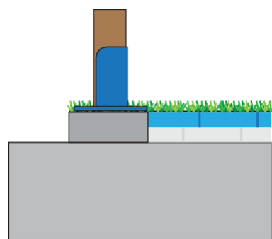
MONTAJE VALLA SOBRE BORDILLO TORNILLOS VISTOS NO ACONSEJABLE
